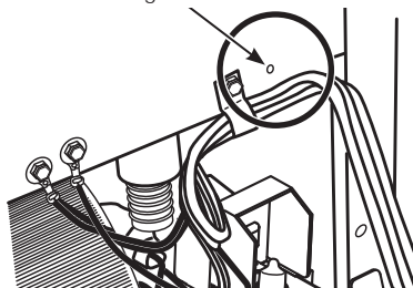
Petit orifice pour l'installation du collier de serrage de la conduite d'eau
